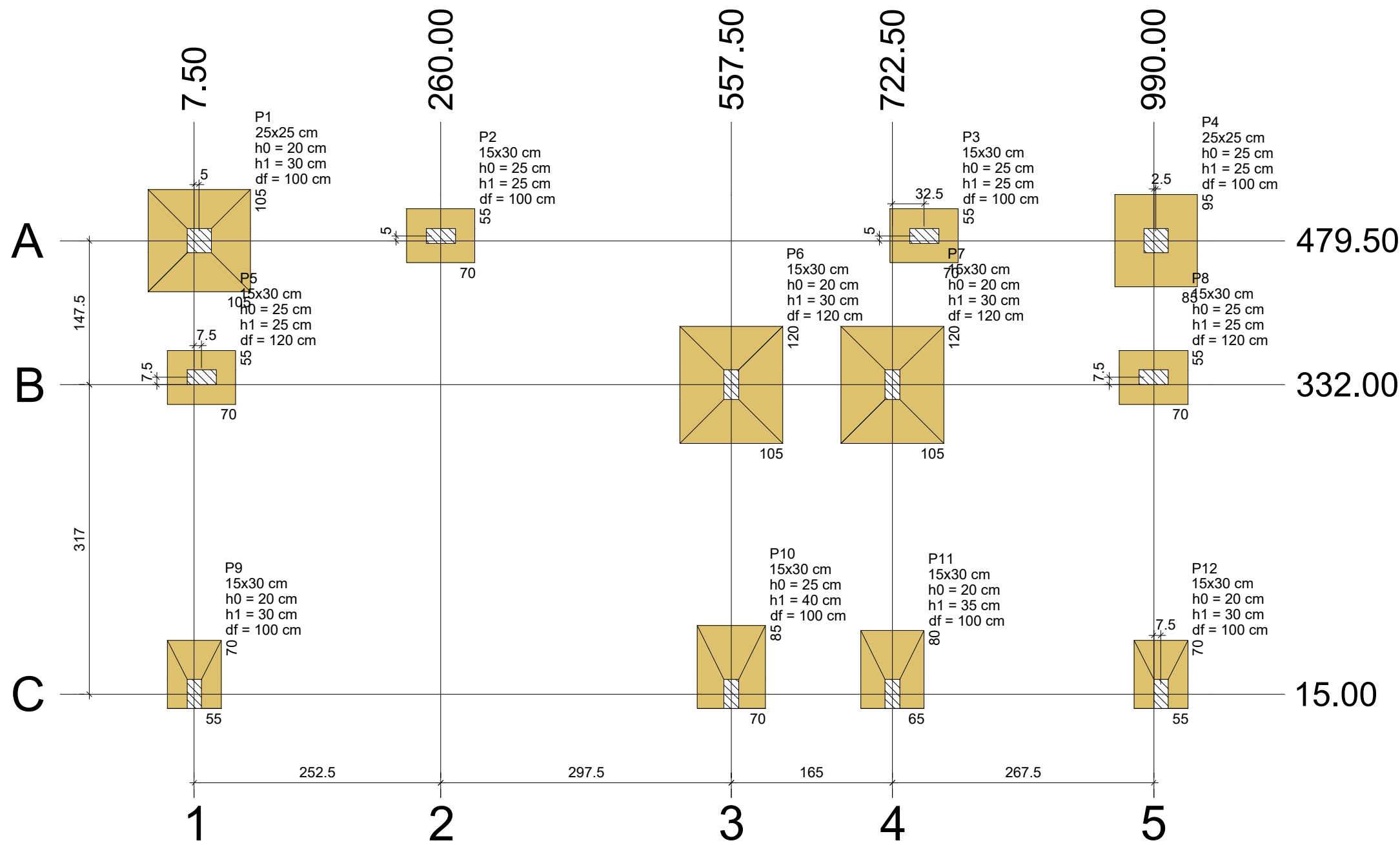
Planta de localização escala 1:50
