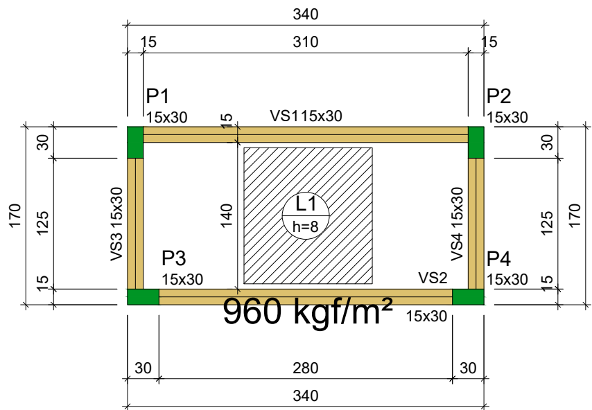
Forma do pavimento +380 (Nível 380) escala 1:50
