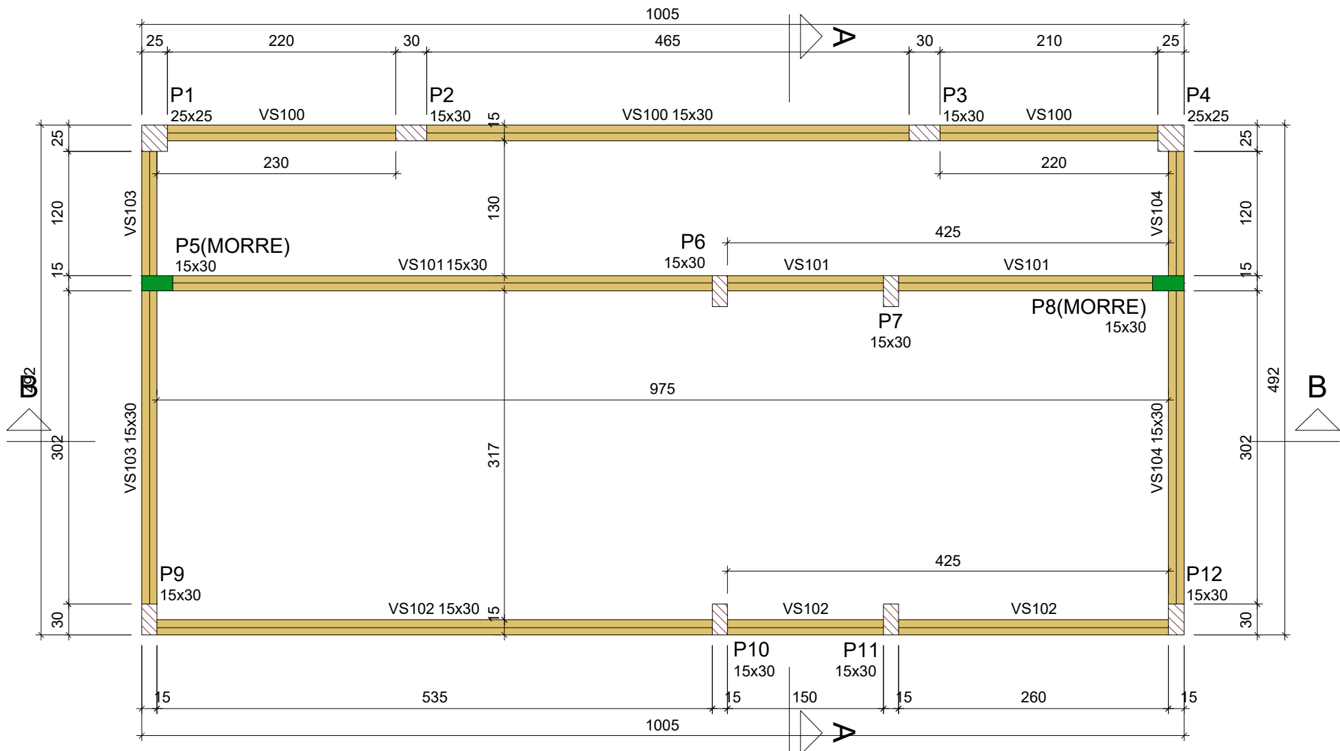
Forma do pavimento +305 (Nível 305) escala 1:50
