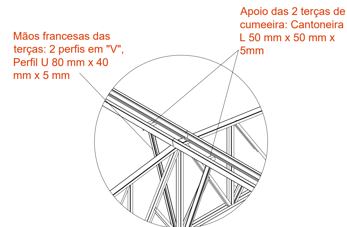
DETALHE DE FIXAÇÃO DAS 2 MÃOS FRANCESAS DAS TERÇAS DE CUMEEIRA S/ ESC
