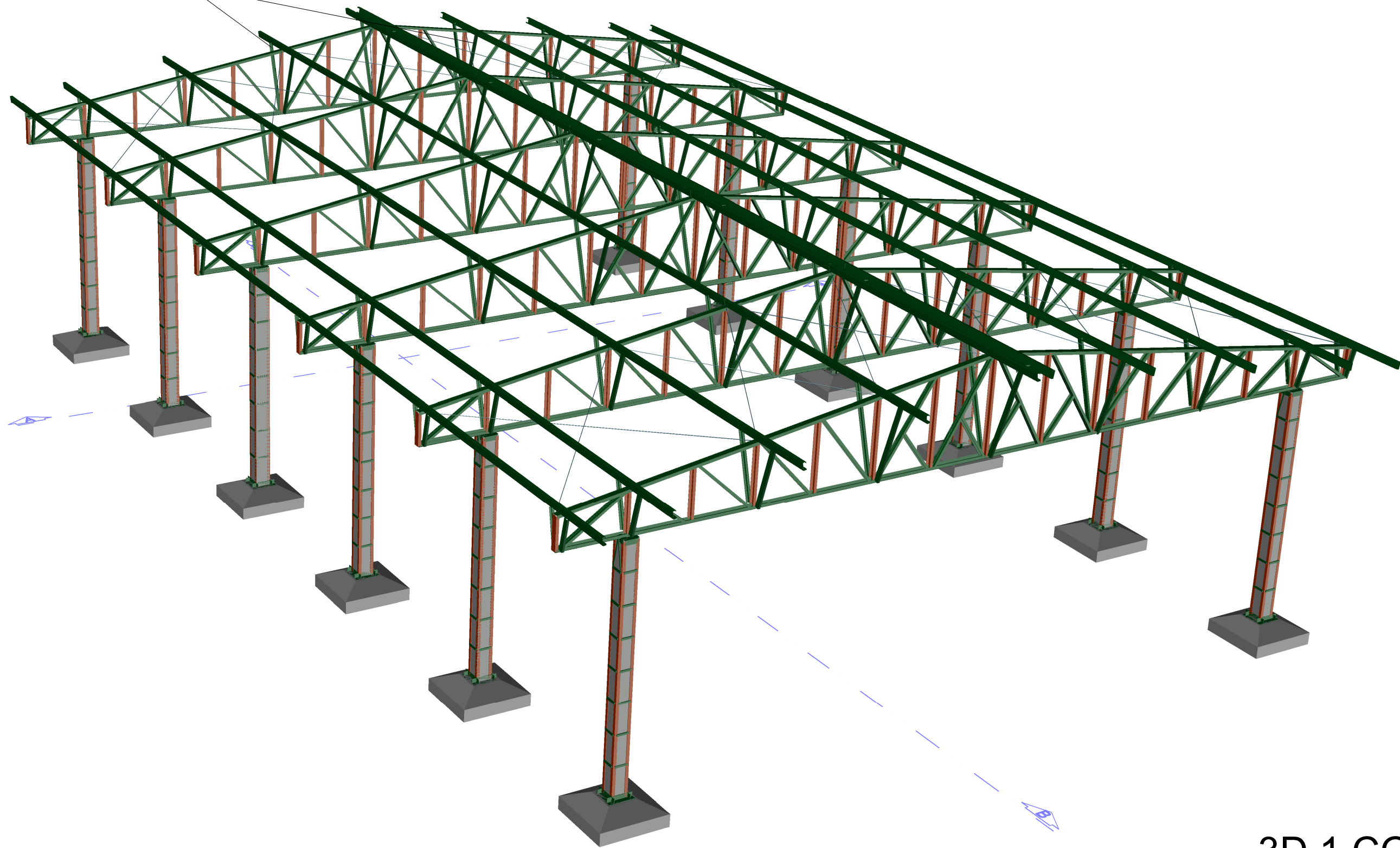
3D 1 COBERTA ESC 1:50
