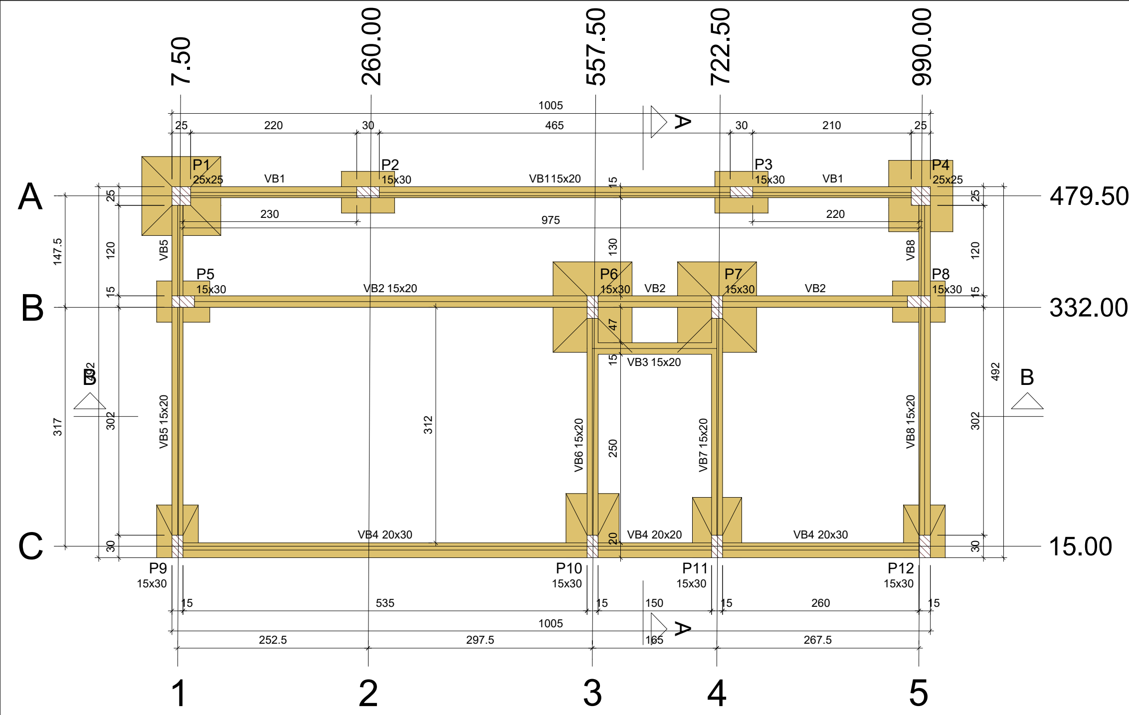
Forma do pavimento +0 (Nível 0) escala 1:50
