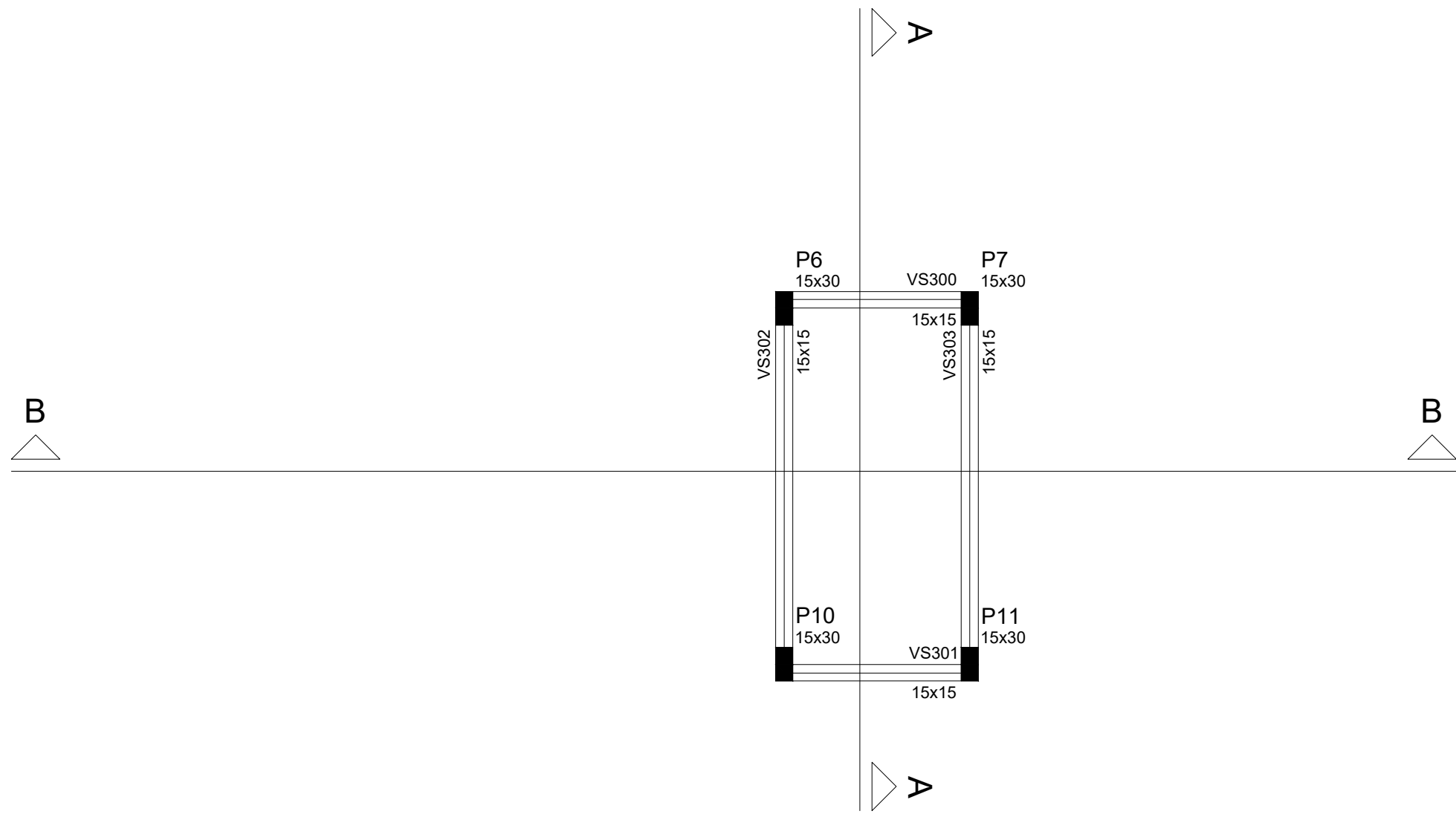
Forma do pavimento +490 escala 1:50
