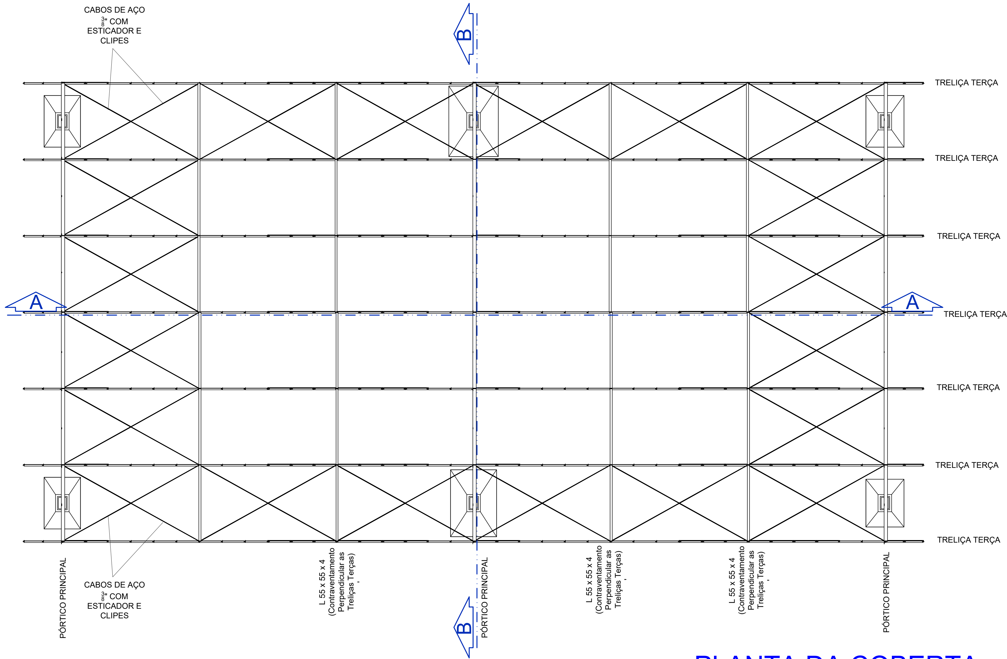
PLANTA DA COBERTA Escala 1/75
