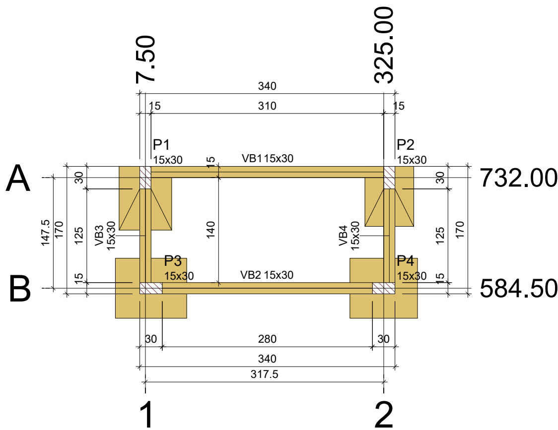
Forma do pavimento +0 (Nível 0) escala 1:50
