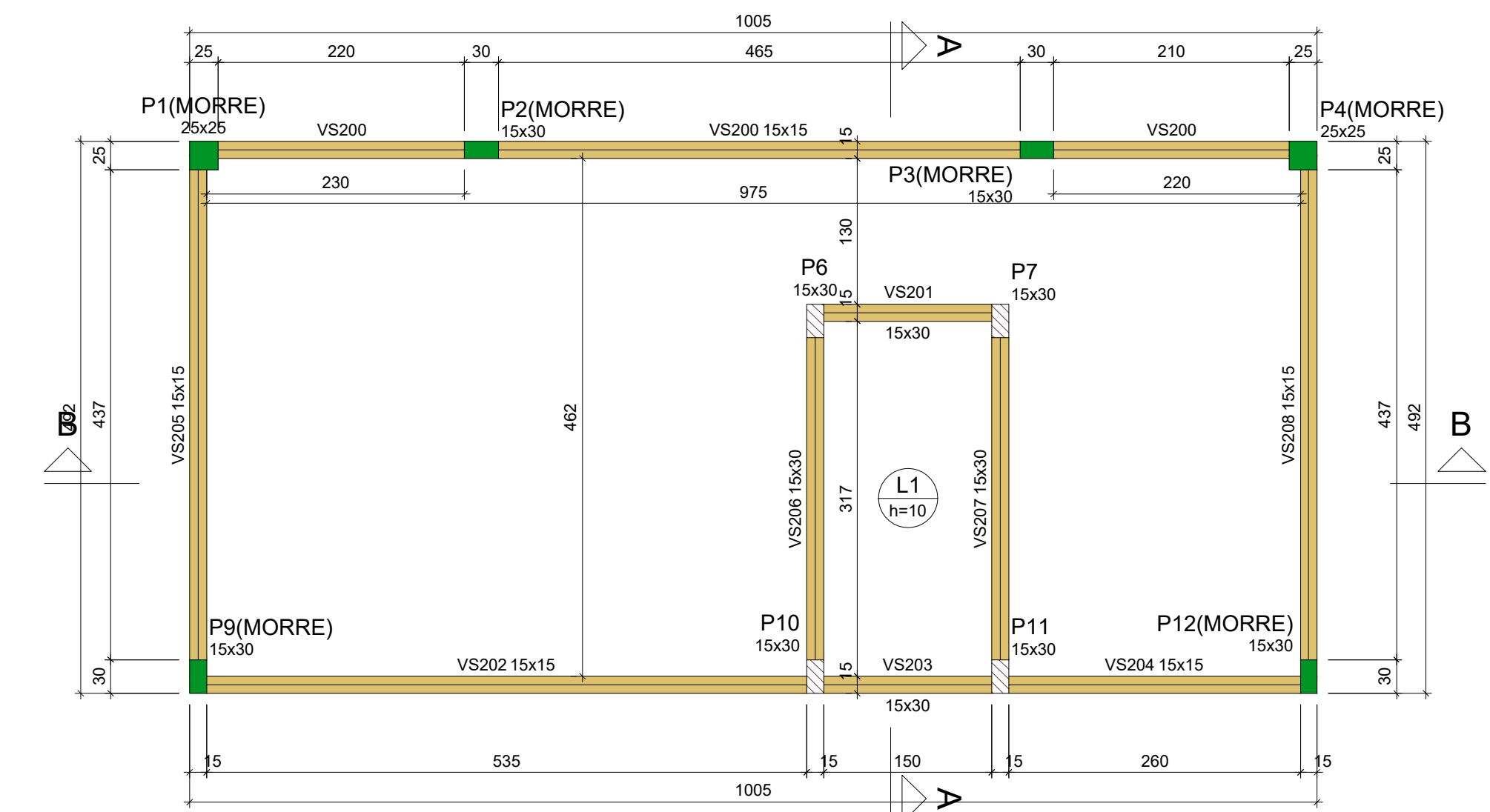
Forma do pavimento +380 (Nível 380) escala 1:50
